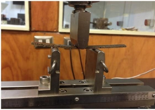
Fig.4:ILSStesting
