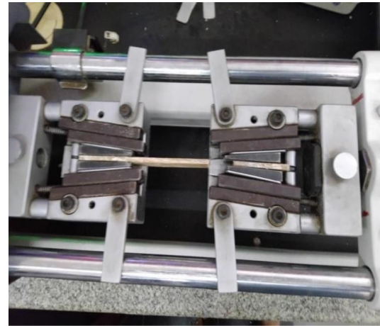
Fig.2: Tensile testing
